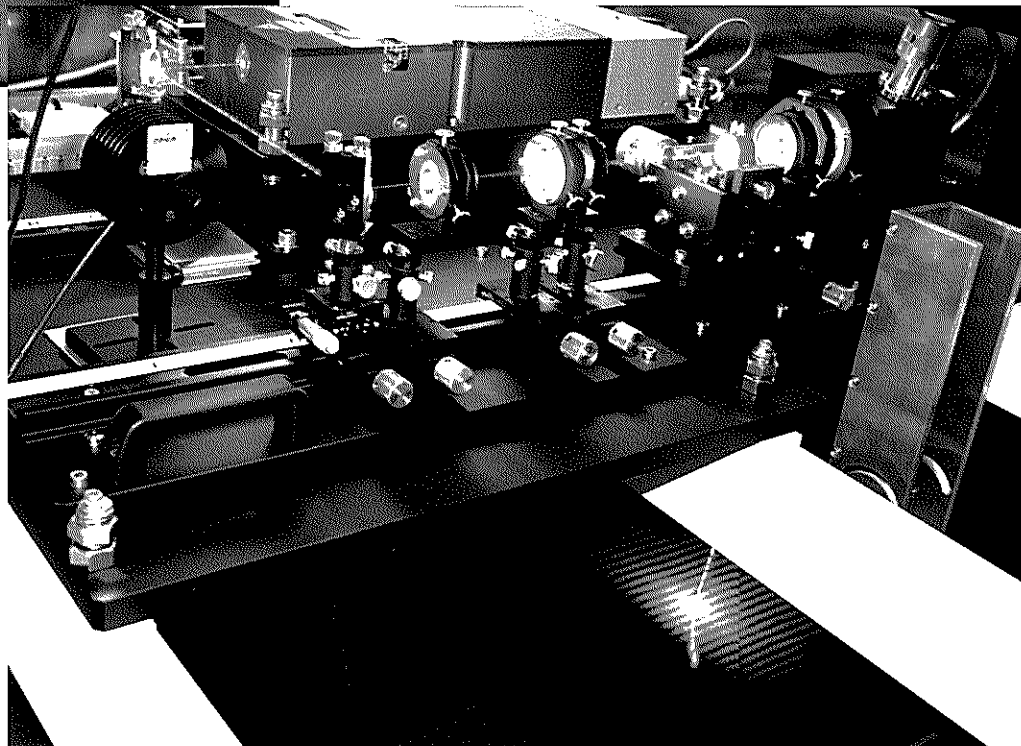
超短パルスレーザーによるCFRPのレーザートリミングのもよう
